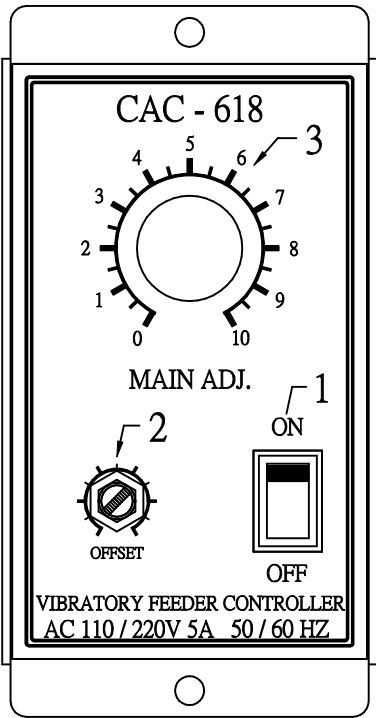
面板配置圖
