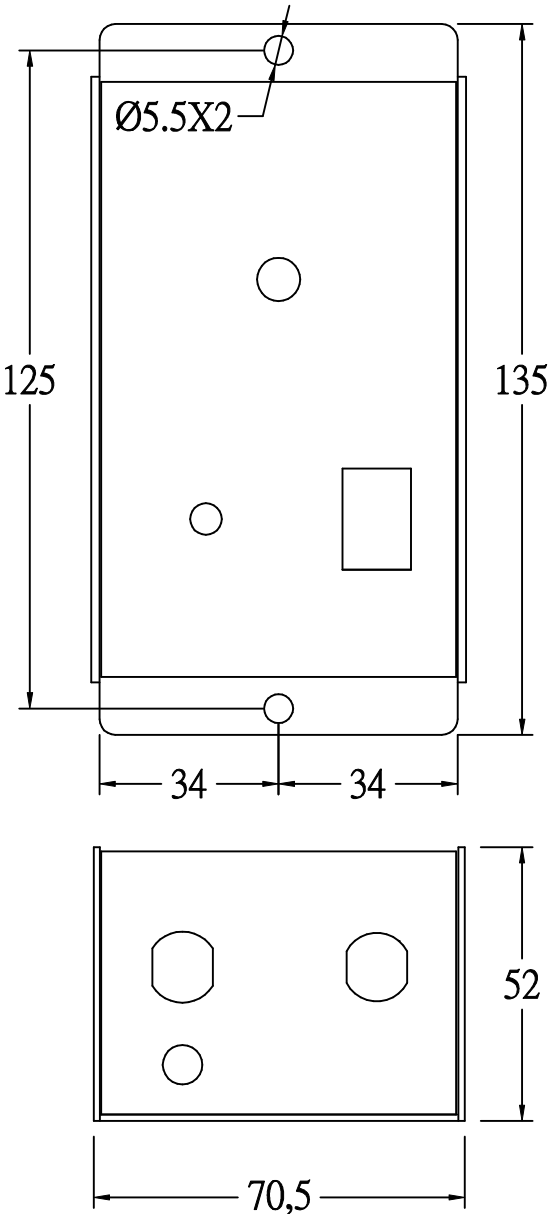
外部尺寸圖
