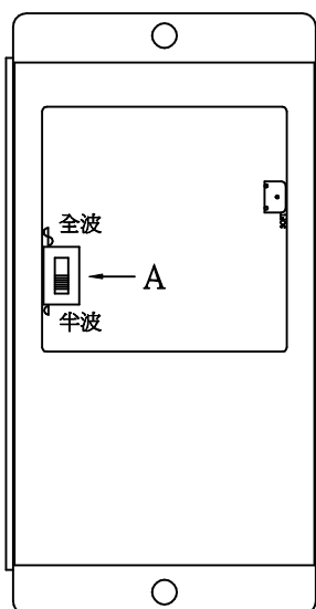
內部配置圖
