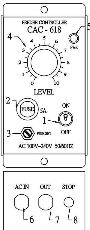
面板配置圖
