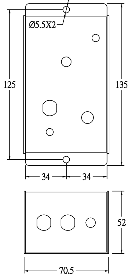
外部尺寸圖
