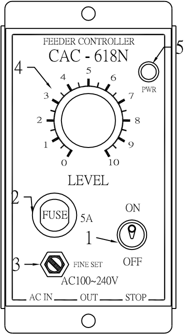
面板配置圖
