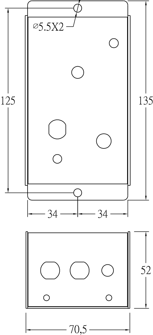
外部尺寸圖
