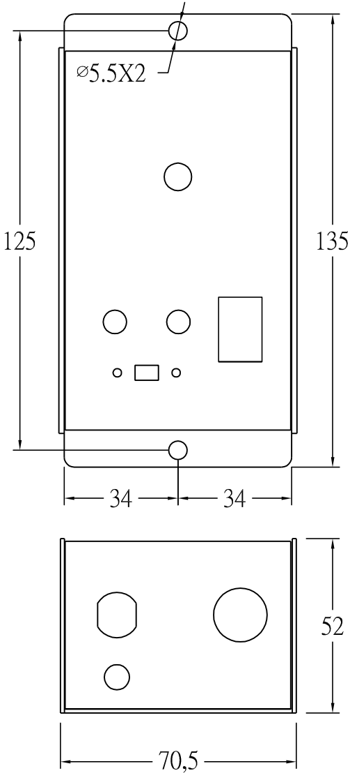
外部尺寸圖
