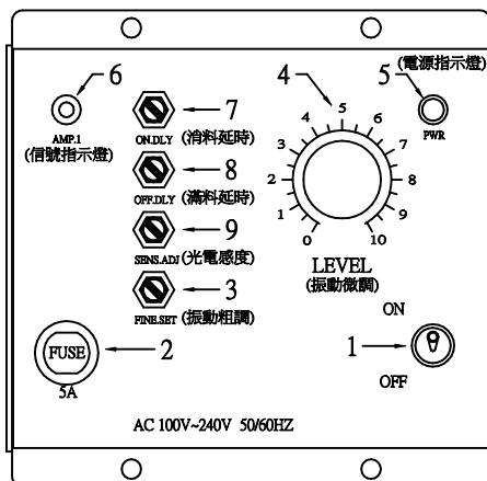
面板配置圖
