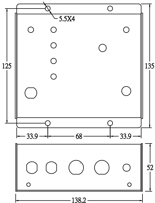
外部尺寸圖
