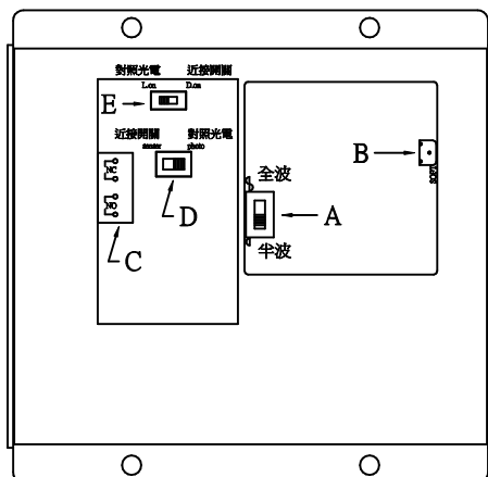
內部配置圖
